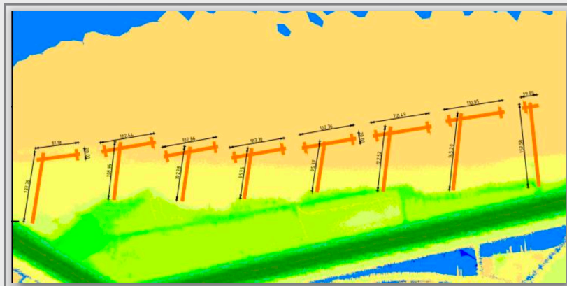
Voorkeursvariant 2a bestaande uit een serie rijshoutdammen voor remming van de golfenergie tijdens jaarrond condities en creëren luwtegebied
